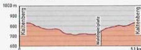
Höhenprofil:
